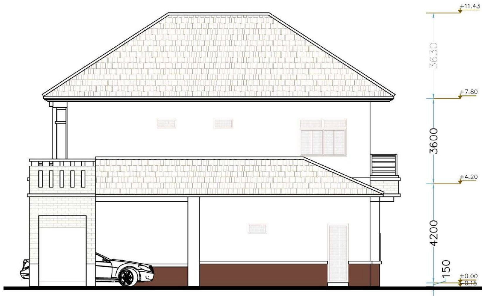
រូបភាពមើលពីខាងស្តាំ RIGHT ELEVATION
