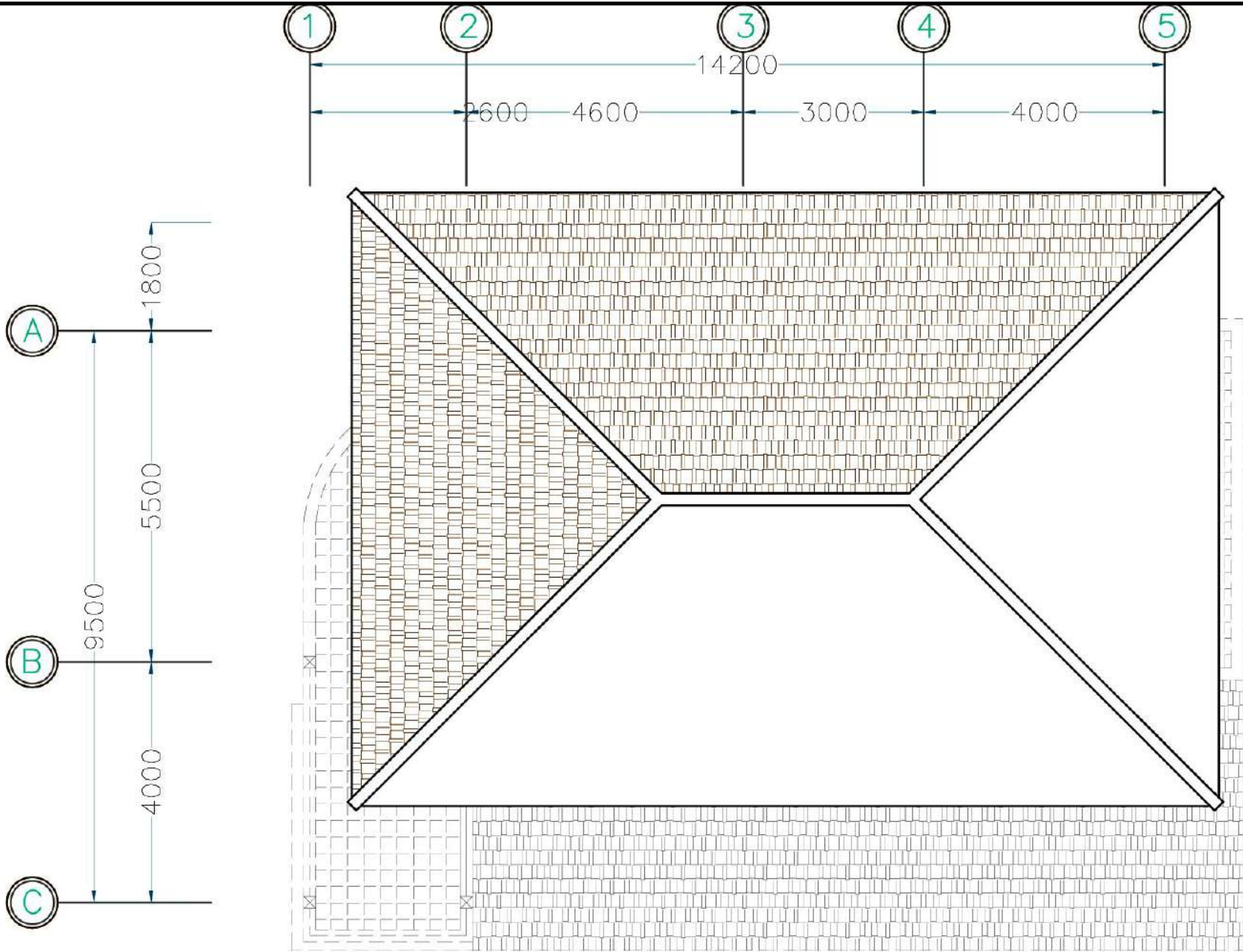
ប្លង់ដំបូល ROOF PLAN
